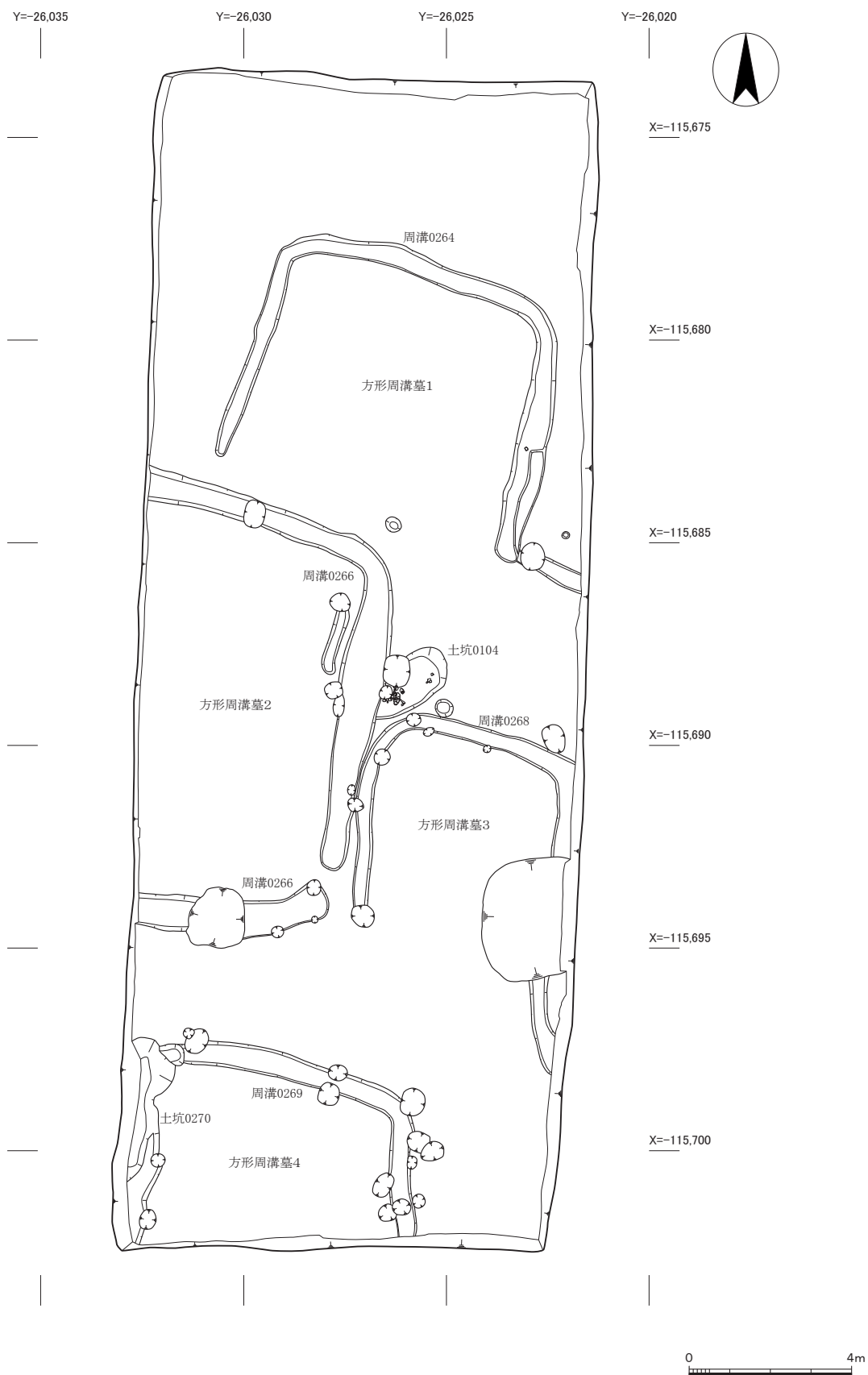
図15 調査区全体平面図（弥生時代）（1：150）
