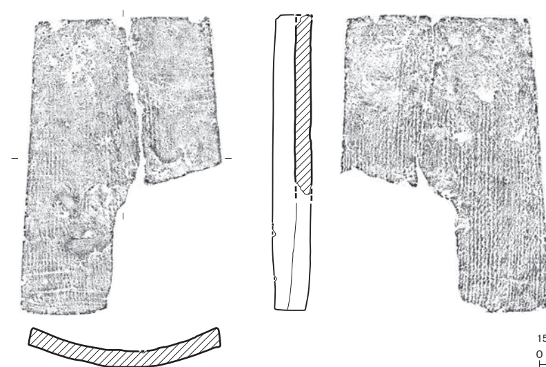
出土瓦類5 (1 : 4)
