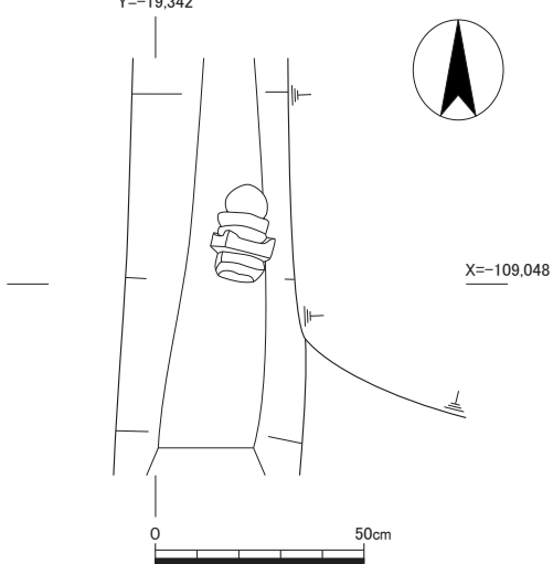
A区沟3·2平面图 (1 : 20、1 : 120)
