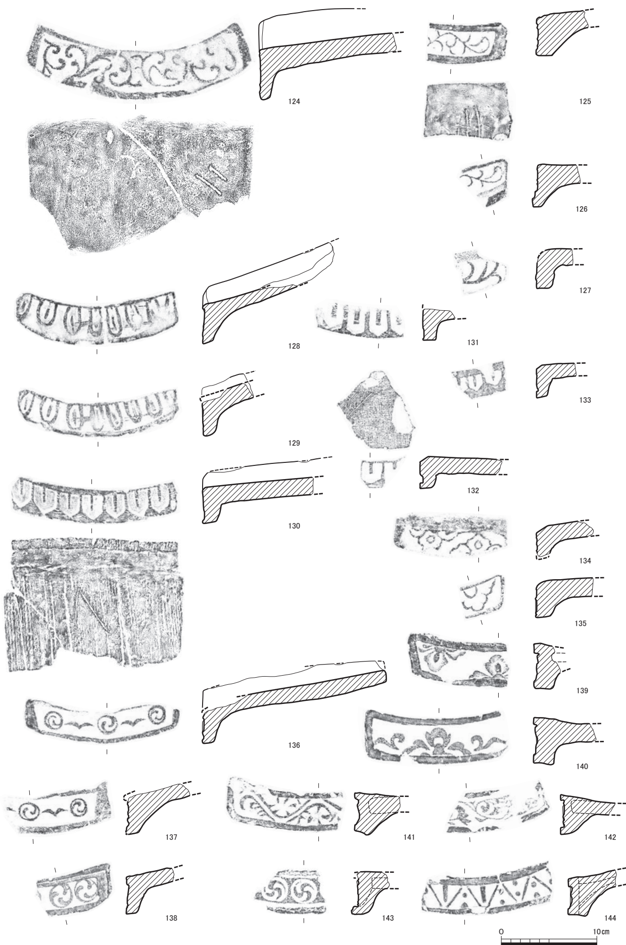
出土瓦類 2 (1 : 4)
