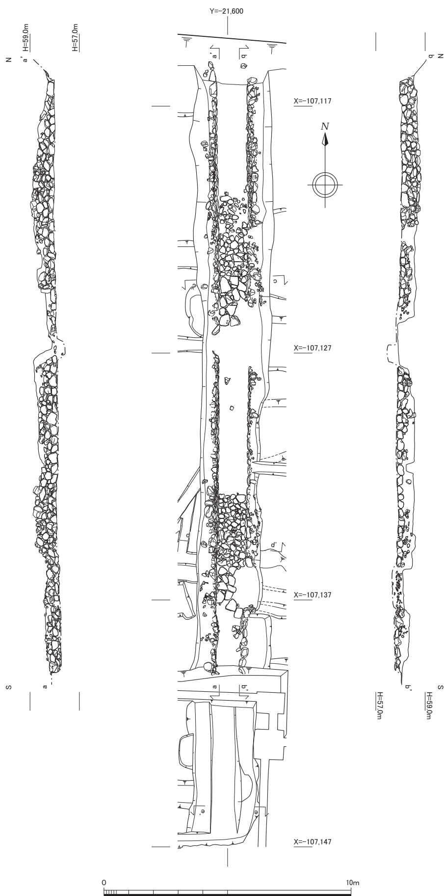
溝0001 平立面図 (1 : 150)
