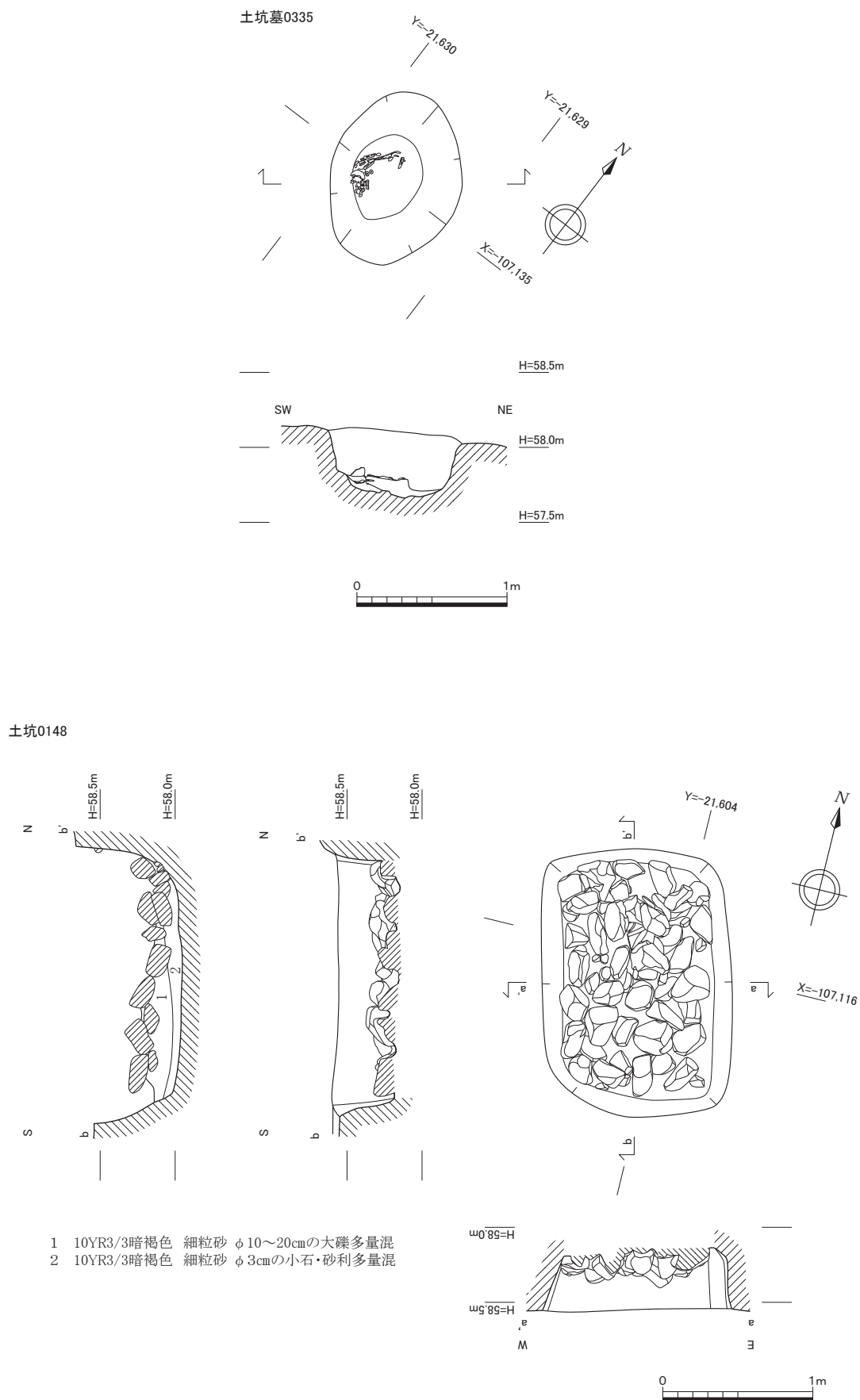
土坑墓0335平断面図（1：40）、土坑0148平断面図（1：40）
