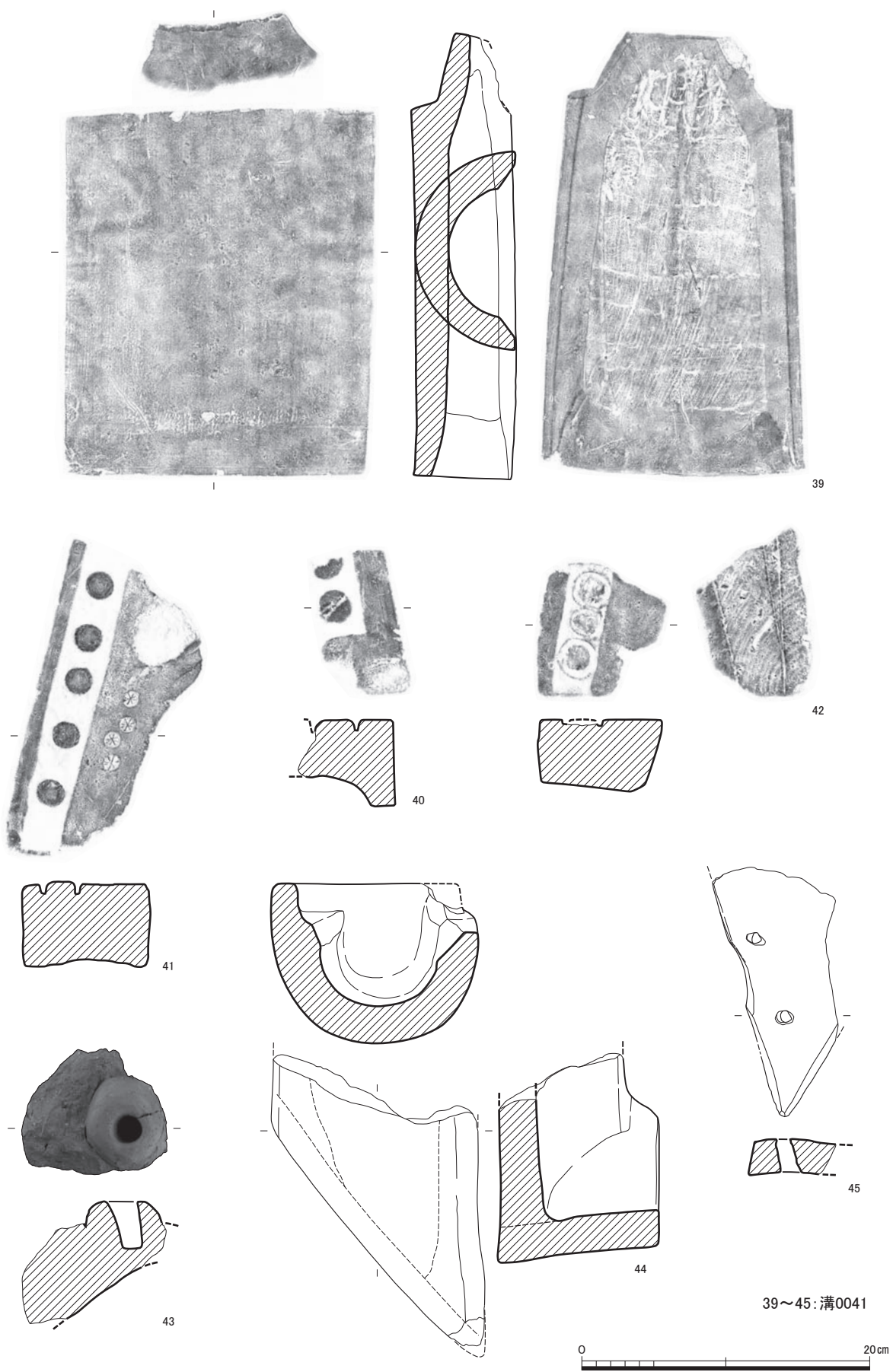
出土遺物5 (1 : 4)
