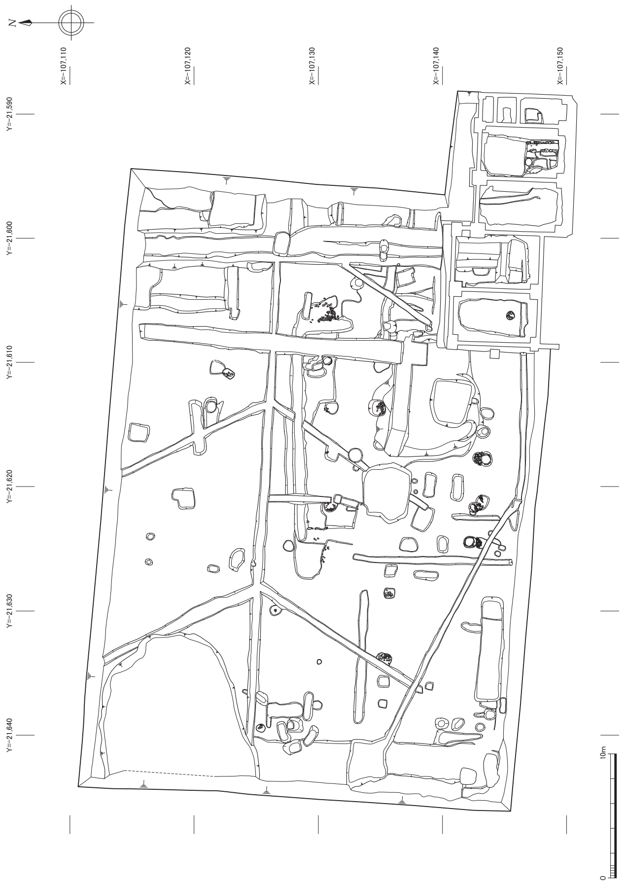
第2-1面 調査区全体平面図 (1 : 300)
