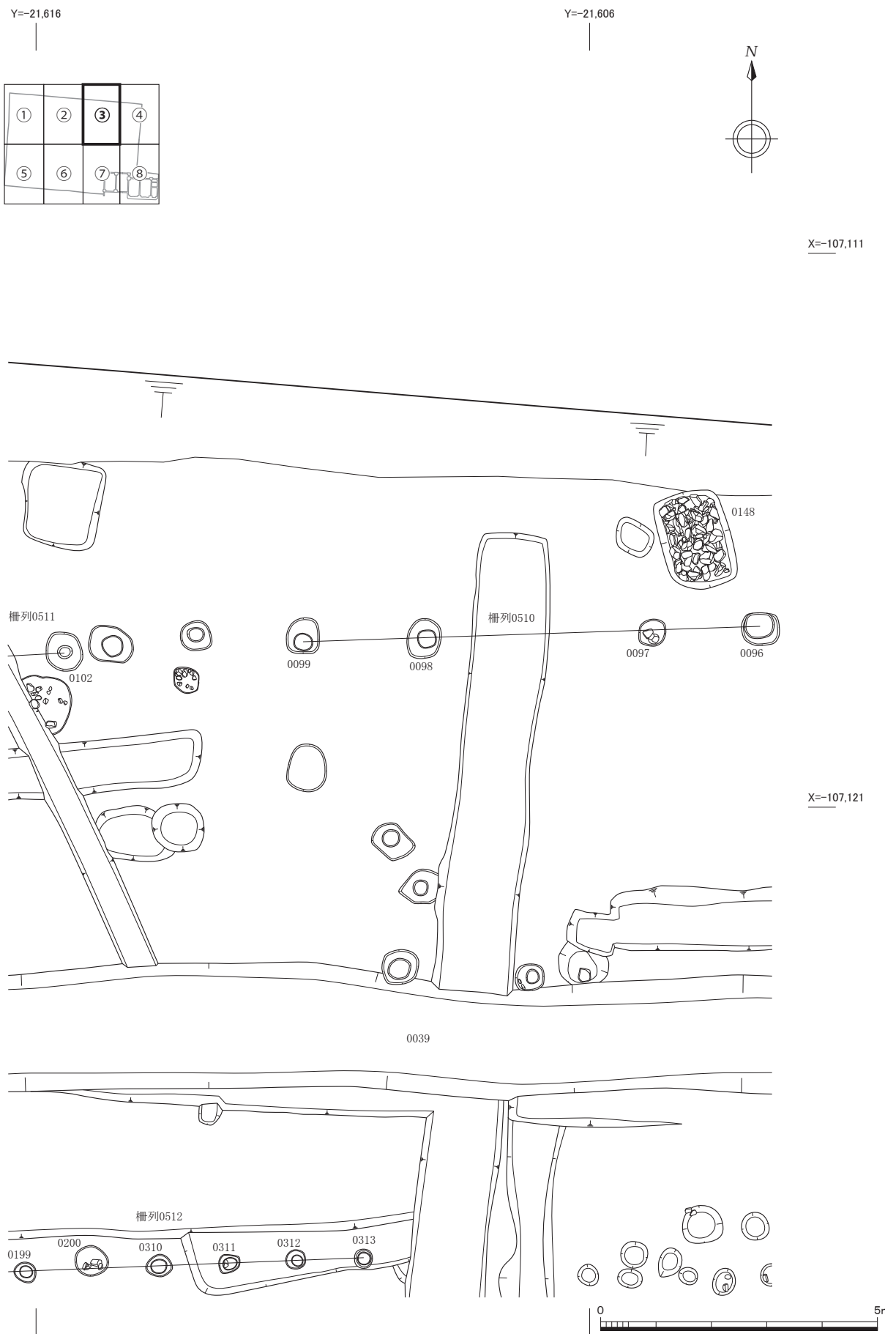
第2-2面 調査区平面図3 (1:100)
