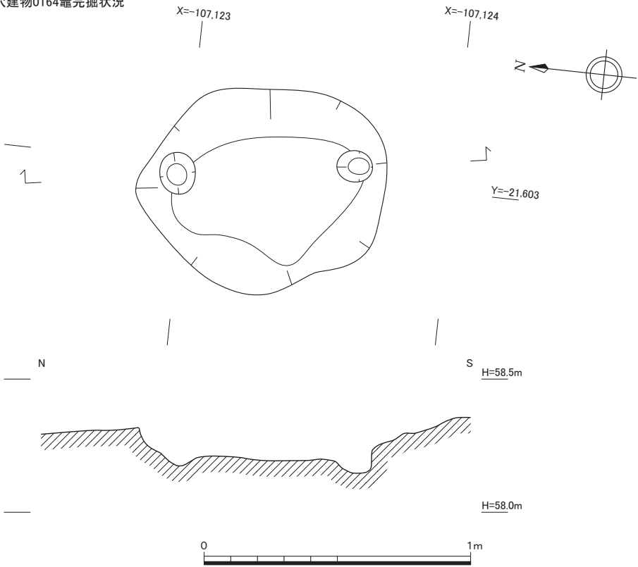
竖穴建物0164竈支柱石検出状況、完掘状況平断面図（1：20）
