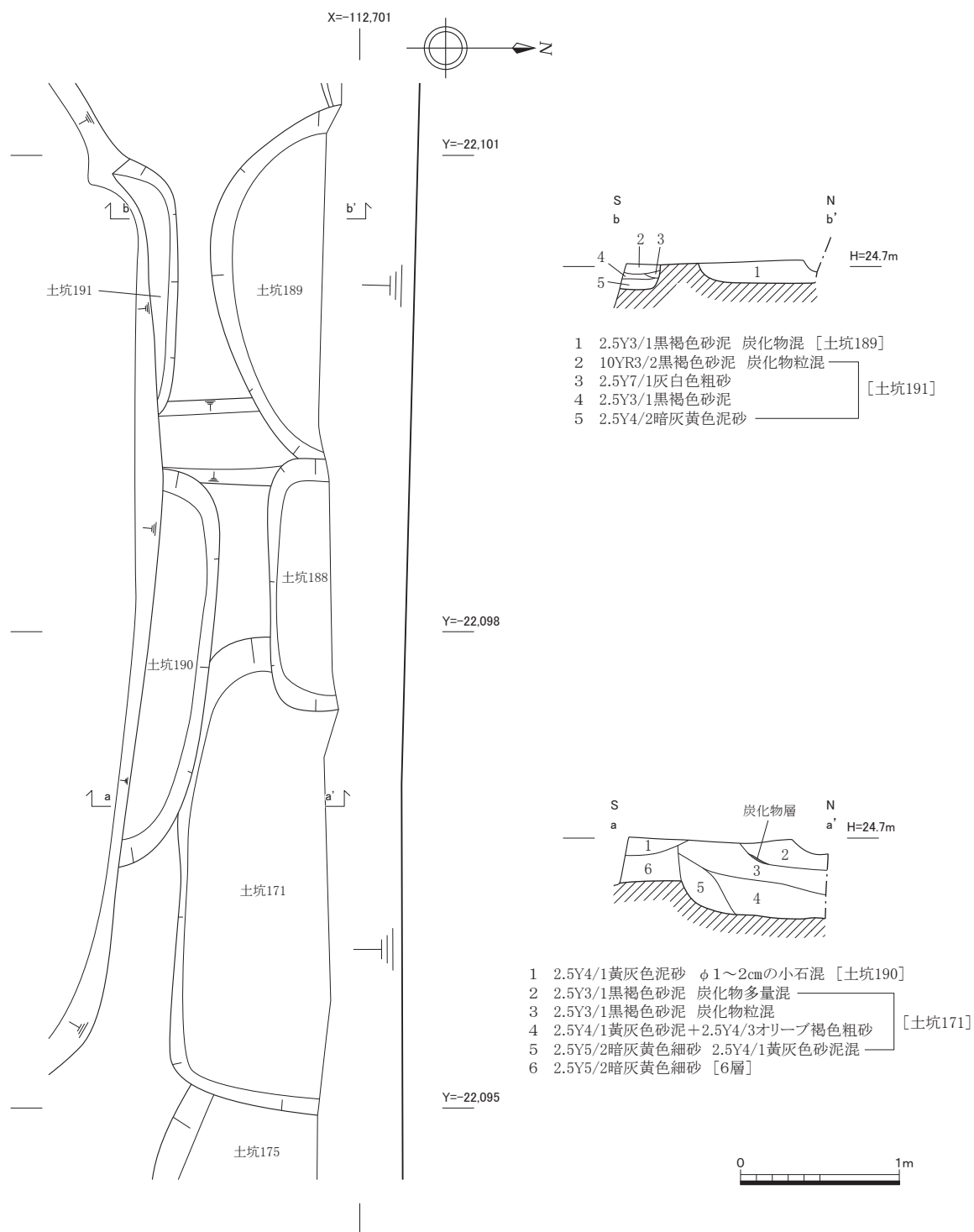
図12 土坑171・190、土坑189・191平面・断面図（1：40）
