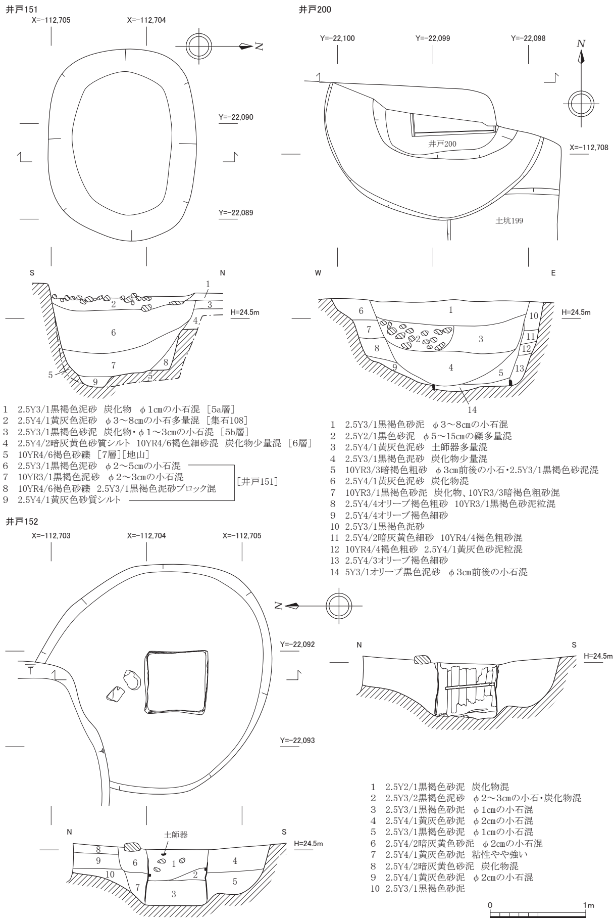
図11 井戸151・152・200平面・断面図 (1:40)
