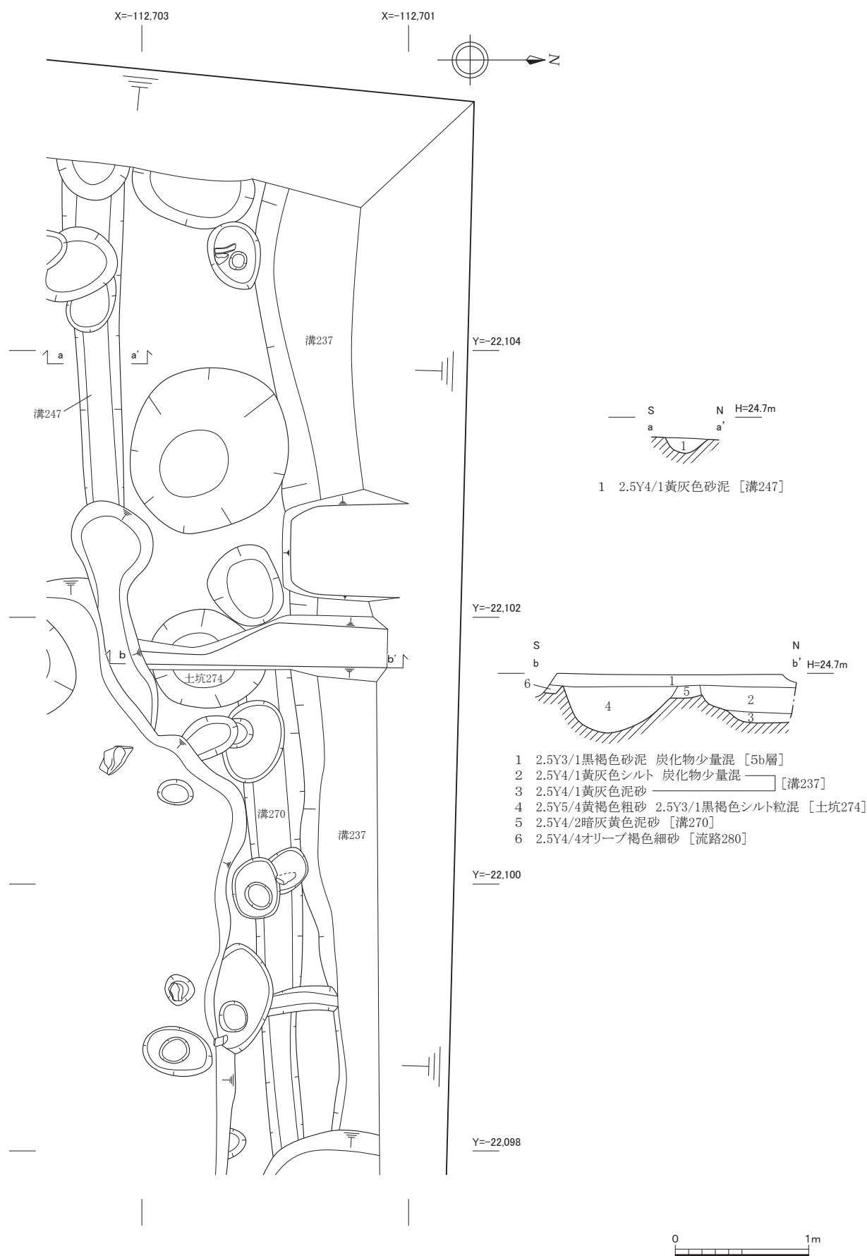
図16 溝247、溝237・270・土坑274平面・断面図（1：40）
