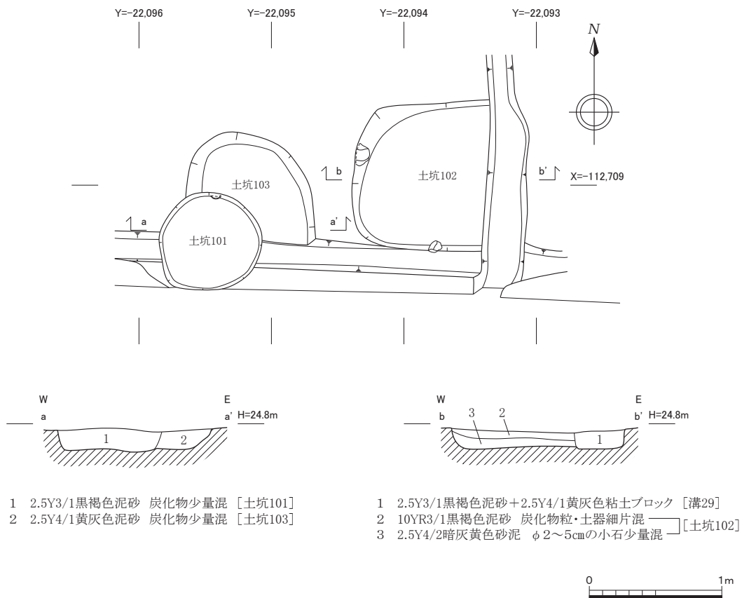
図9 柱列140、土坑101・102・103平面・断面図（1：40）
