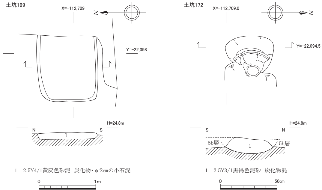
図13 土坑199・172平面・断面図（土坑199 1:40、土坑172 1:20）
