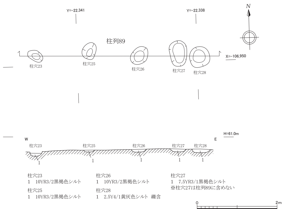
図18 柱列89平面・断面図（1：50）
