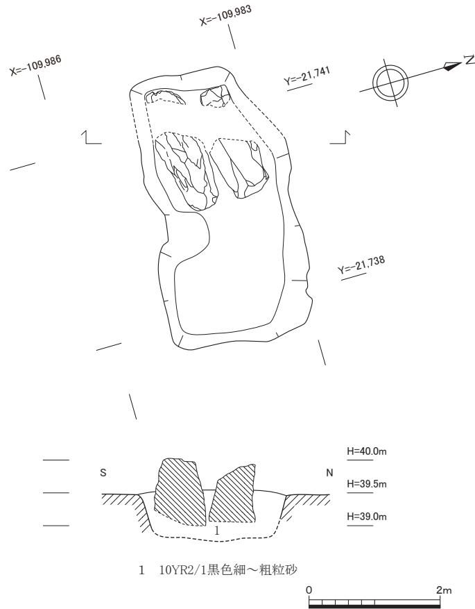
礎石列0368平・断面図（1：40）、土坑0007平・断面図（1：80）
