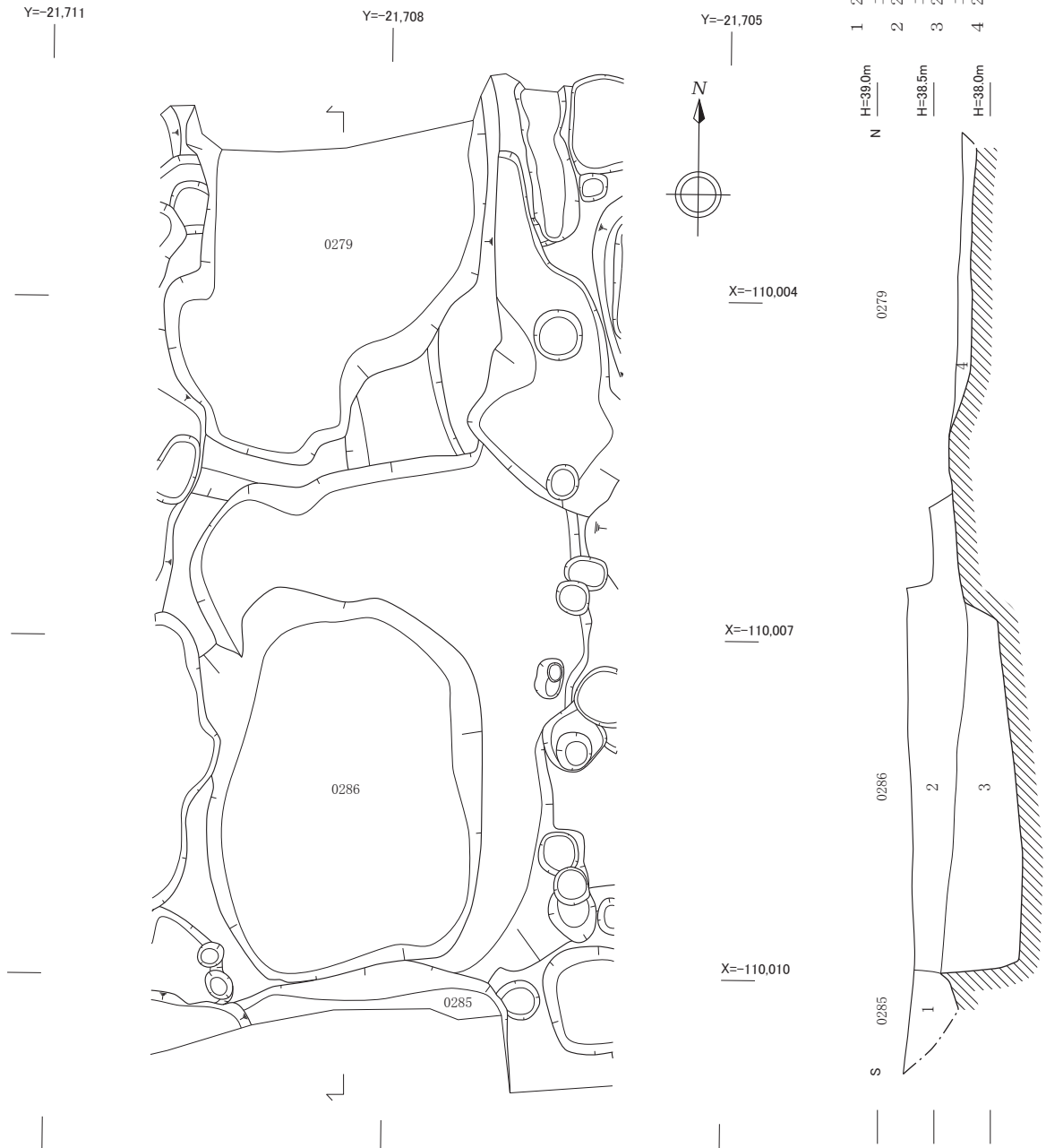
土坑0279・0286・0285平・断面図（1：60）
