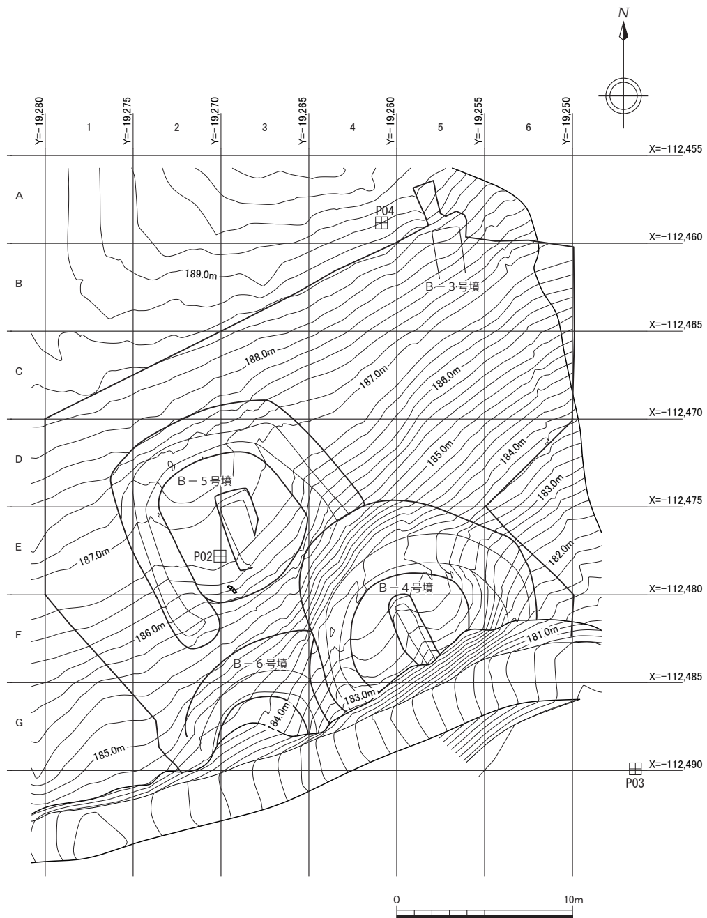
図3 調査区地区割・基準点配置図 (1:200)
