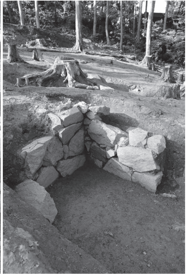
2. B-5号墳 石室左側壁構築状況 (南西から)
