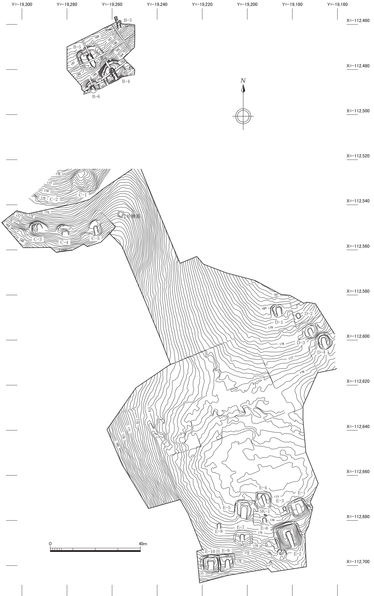
B~E支群合成平面図 (1 : 1,000)
