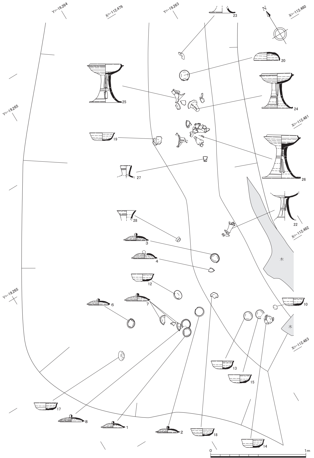
B-4号墳周溝内遺物出土状況平面図 (1:20)
