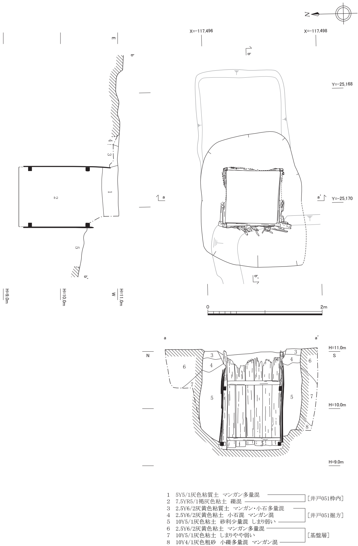
図16 東区 井戸051 平断立面図 (1 : 40)
